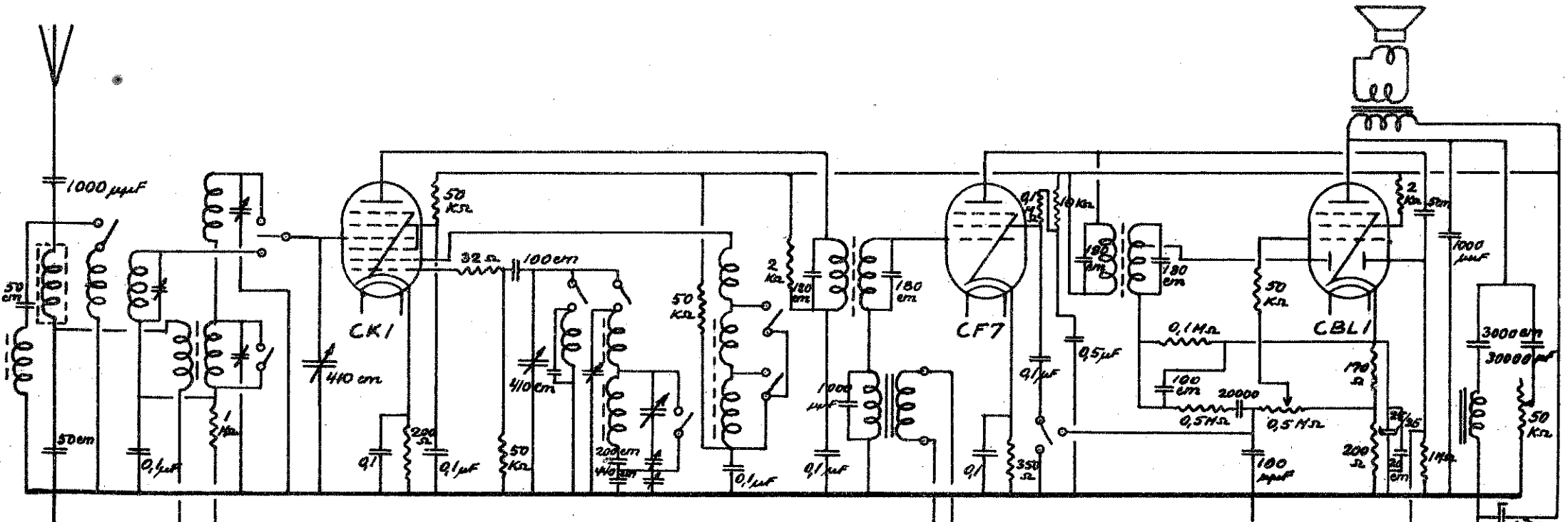
Omskifter.
