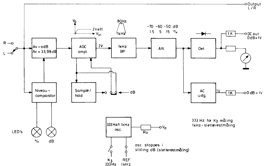
(Fig. 7 blokdiagram)
