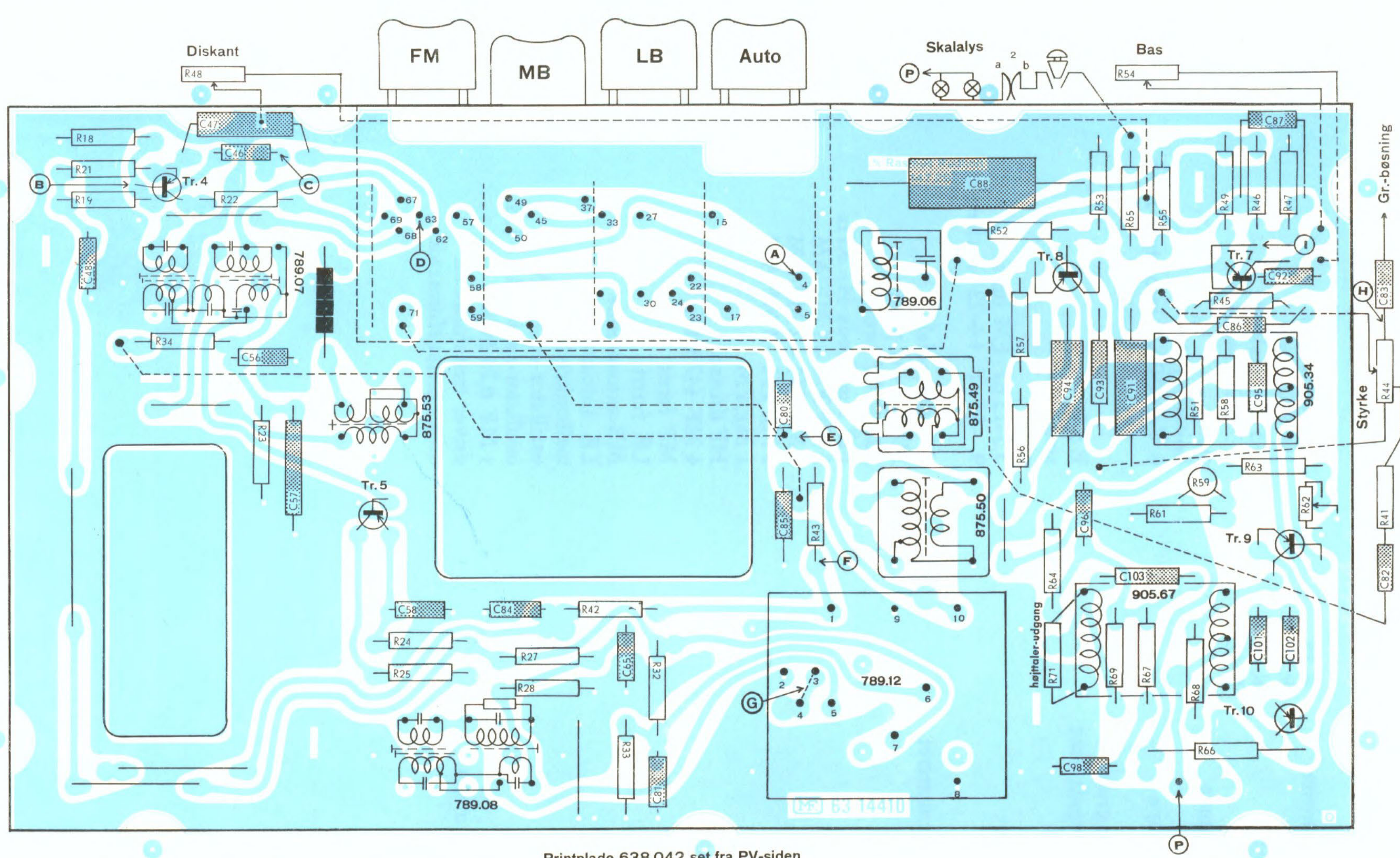
Printplade 638.042 set fra PV-siden
